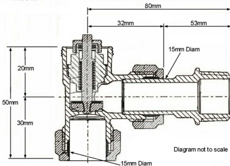
TRV2 BODY
